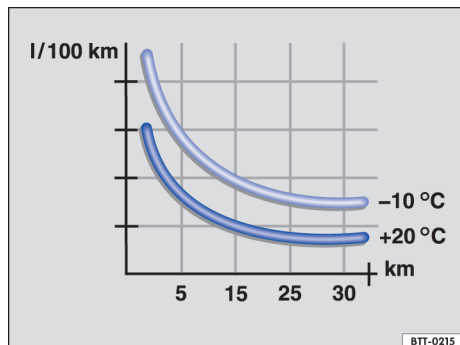
图 84 两种不同环境温度时的百公里油耗 (l/100km)。
