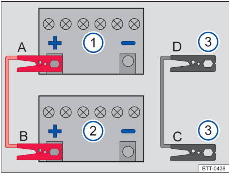
图 130 连接起动辅助电缆的示意图
