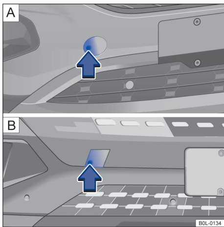
图 133 前保险杠上右侧：取下盖板
