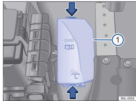
图 127 发动机舱内：保险丝盒的盖板 ①。
