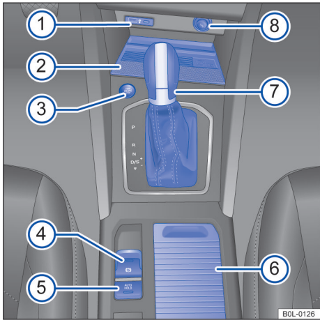
图 9 中控台下部概貌
