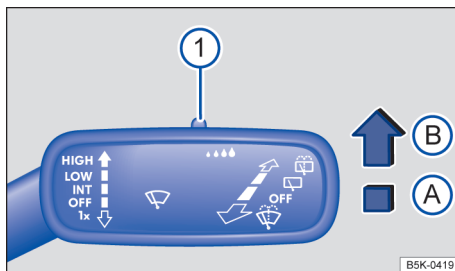
图 73 转向柱右侧：风窗刮水器操纵杆
