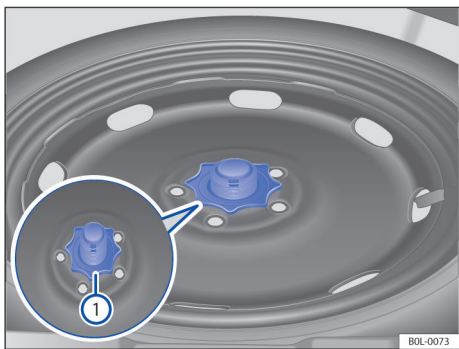
图 157 在行李箱内：用于固定应急备用车轮的手轮；
