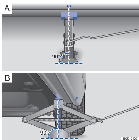
图 159 千斤顶放置在车辆左侧后部
