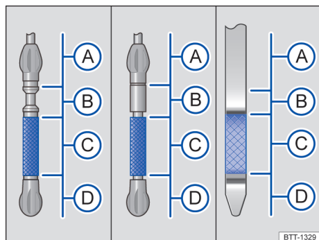
图 140 带机油油位标记的机油标尺（示例）
