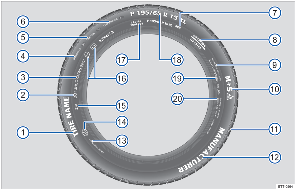
图 153 国际通用轮胎识别字母
