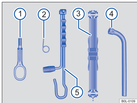
图 122 交货范围所含工具
