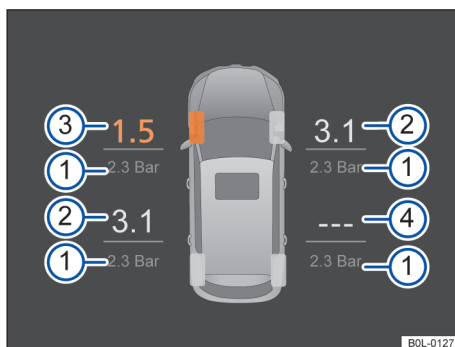
图 148 组合仪表显示屏显示：当前胎压
