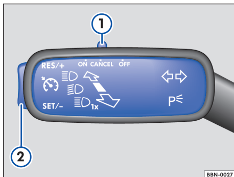
图 94 转向柱左侧：操作 GRA 的开关和按钮
