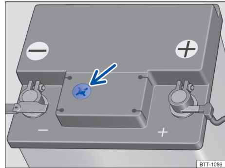
图 145 12 伏车载蓄电池上侧的蓄电池观测孔（示意图）
