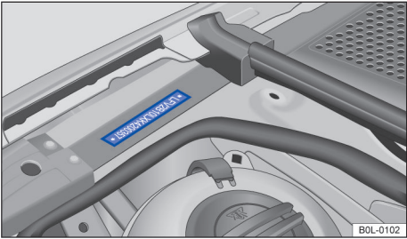
图 165 发动舱内：车辆识别代号（示意图）
