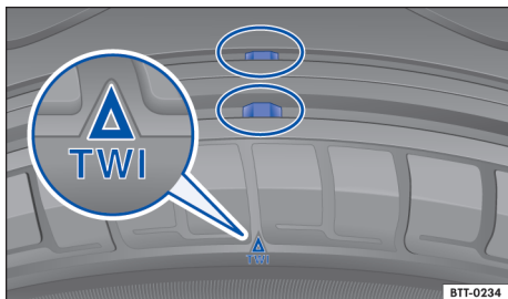
图 152 轮胎花纹：磨损标记（示意图）
