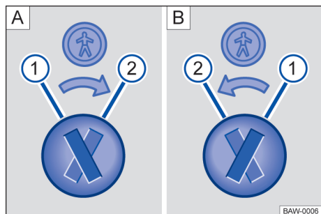
图 50 儿童安全门锁：A 左后车门，B 右后车门
