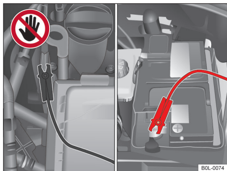
图 146 发动机舱：充电装置或辅助启动电缆的接口
